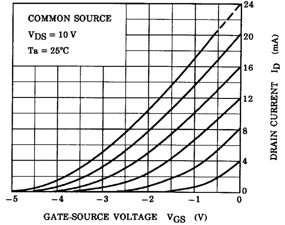
ID - VGS
