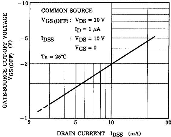
VGS(OFF) - IDSS
