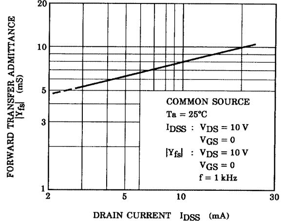
|Yfs| - IDSS
